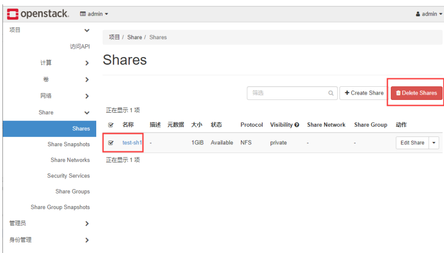
图 4-3 删除共享
