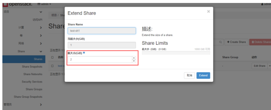
图 4-6 共享扩容
